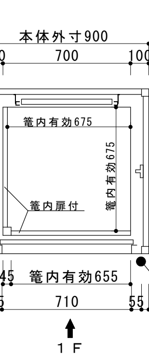
升降路平面図 1/20
