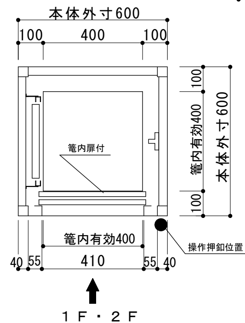
升降路平面図 1/15
