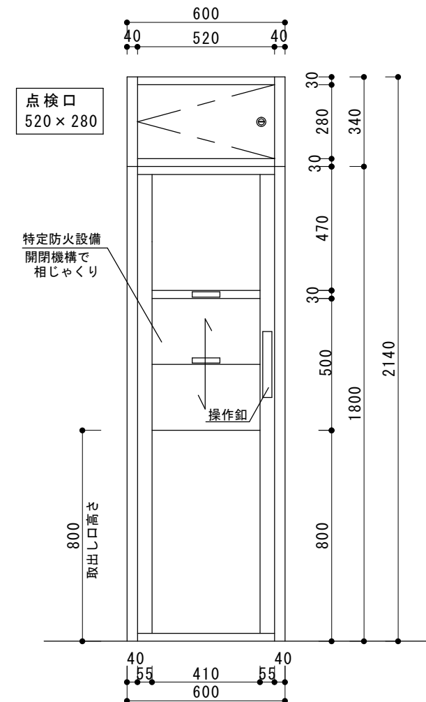
2階立面図 1/20
