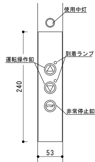
操作釦 1/5
