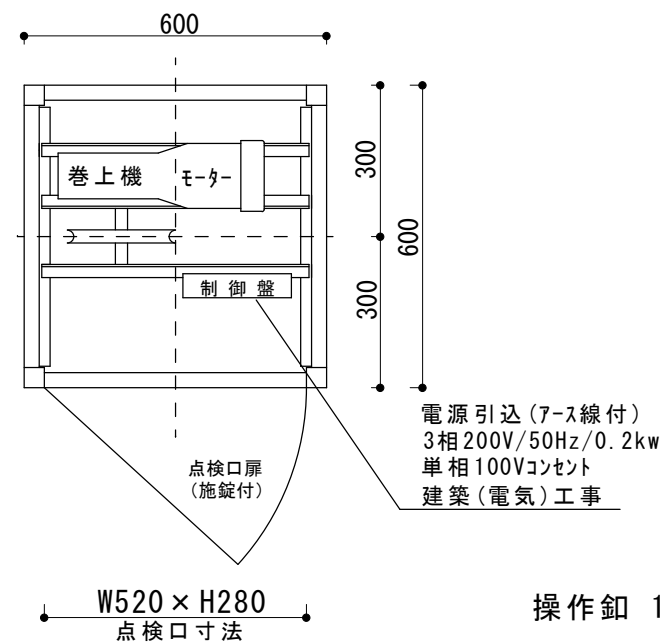
機械室平面図 1/15
